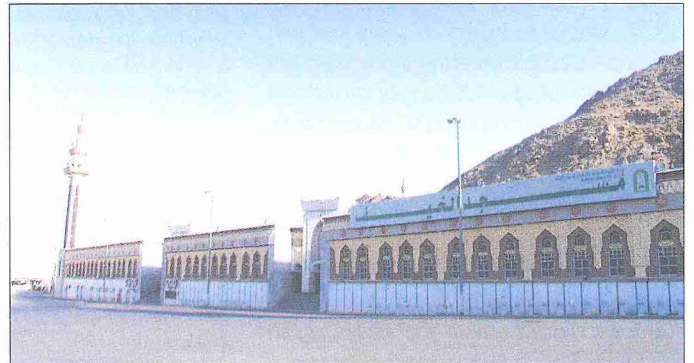
Mescid-i Hayf
